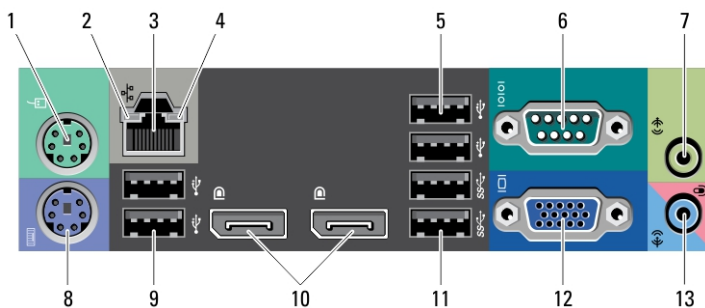
Figura 2. Vista do painel traseiro da minitorre
