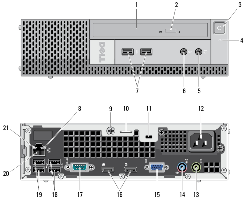
Figura 5. Visão frontal e traseira do fator de forma ultra pequeno
