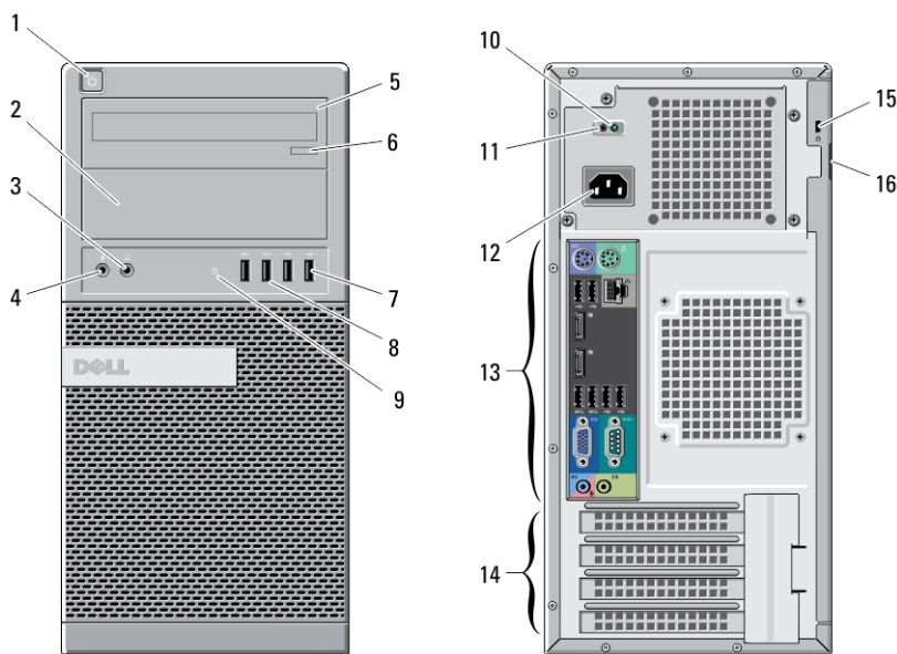
Figura 1. Visão dianteira e traseira da minitorre
