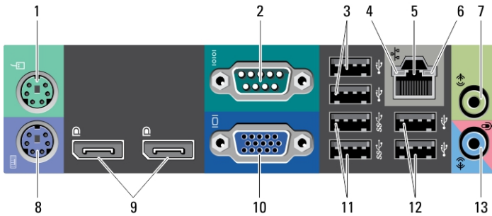
Figura 4. Visão do painel traseiro do fator de forma pequeno
